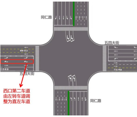
▲五四大街与同仁路交叉口交通组织优化示意图
