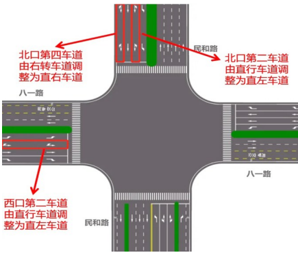
▲八一路与民和路交口交通组织优化示意图
