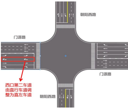
▲朝阳西路与门源路交叉口交通组织优化示意图
