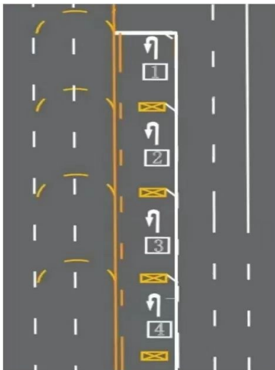
柴达木路石油小区西口设置联动式掉头示意图。
