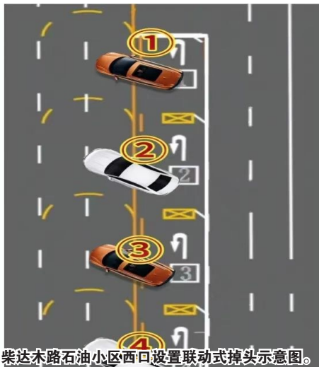
柴达木路石油小区西口设置联动式掉头示意图。
